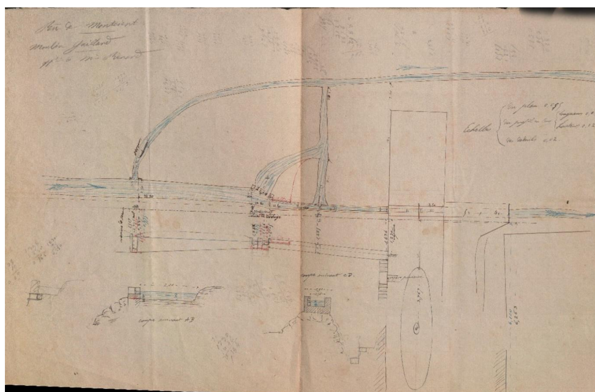
Plan des eaux alimentant le moulin Gaillard fourni par Eustache RENARD pour la modification du déversoir (archives départementales des Yvelines, 7S 180).
