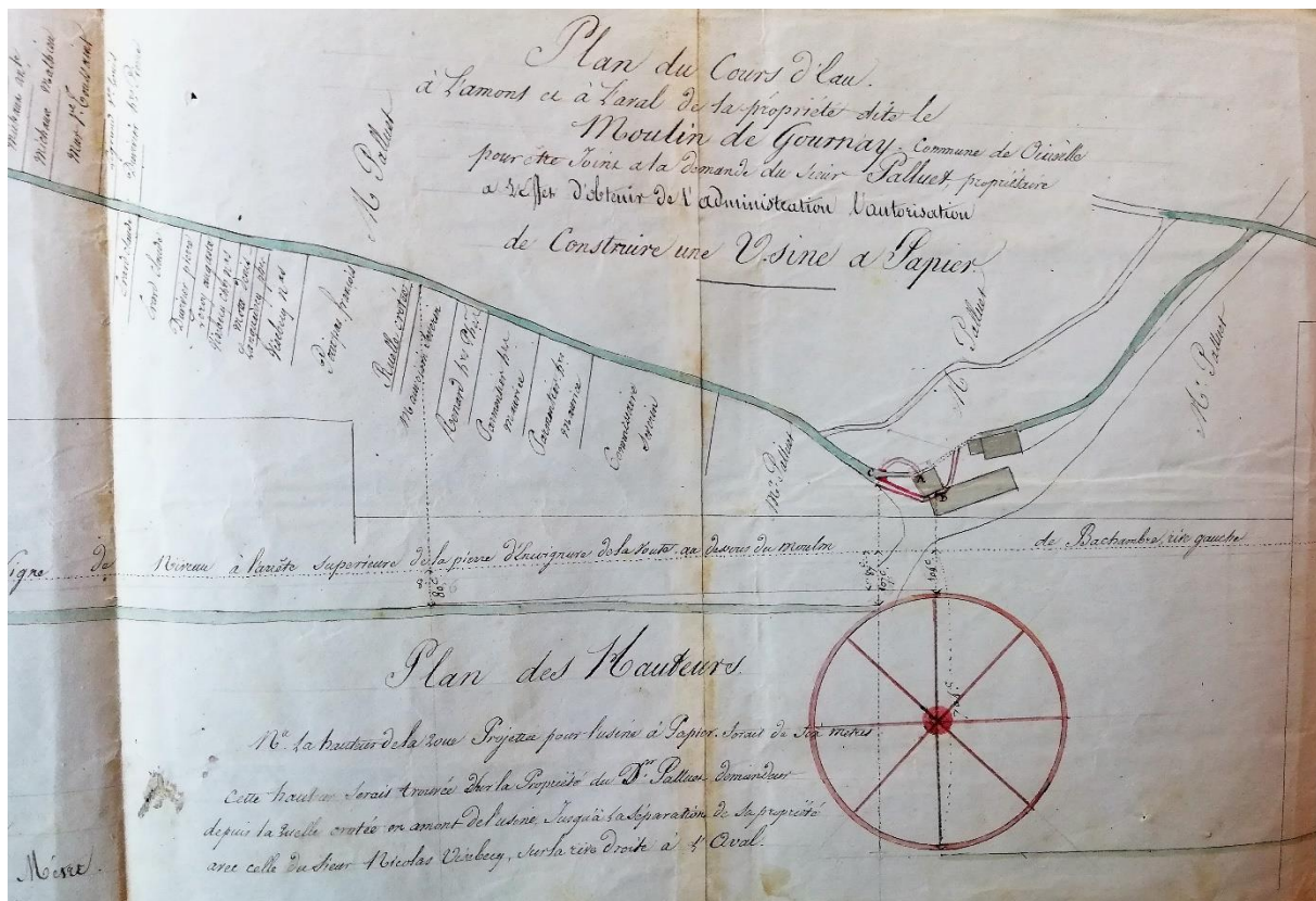
Plan du cours d'eau en amont et en aval de la propriété dite du moulin de Gournay commune de Oinville pour être joint à la demande du Sieur PALLUET propriétaire à l'effet d'obtenir l'autorisation de l'administration de construire une usine à papier (extrait du plan et détail).
